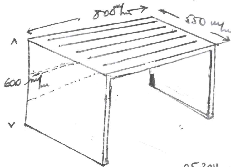
SOPORTE MALETA
